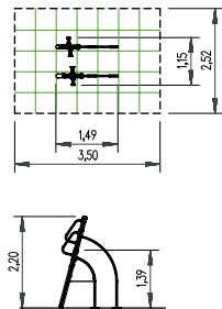
5 54 010 0 eibe fit Aktiv-Station Leg massage 1:100
