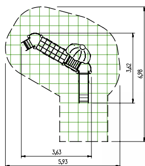
5 59 838 5 eibe minimondo Coral 1:200
