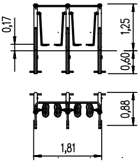
5 54 002 0 eibe fit Aktiv-Station leg trainer 1:100
